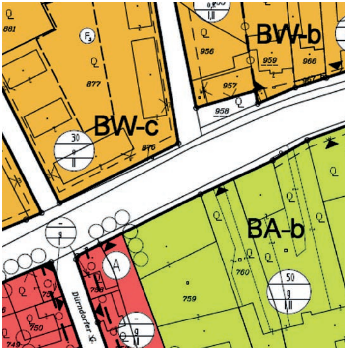
Beispiel Bebauungsplan
